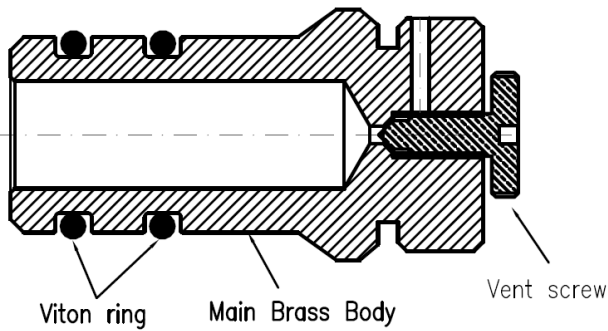
Air vent
